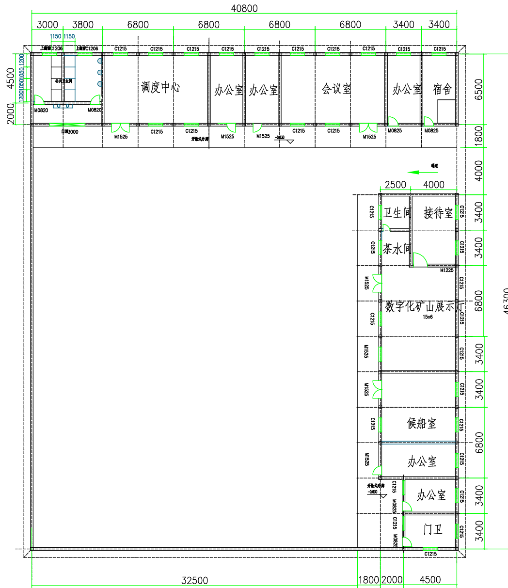
进岛广场用房平面布置图
